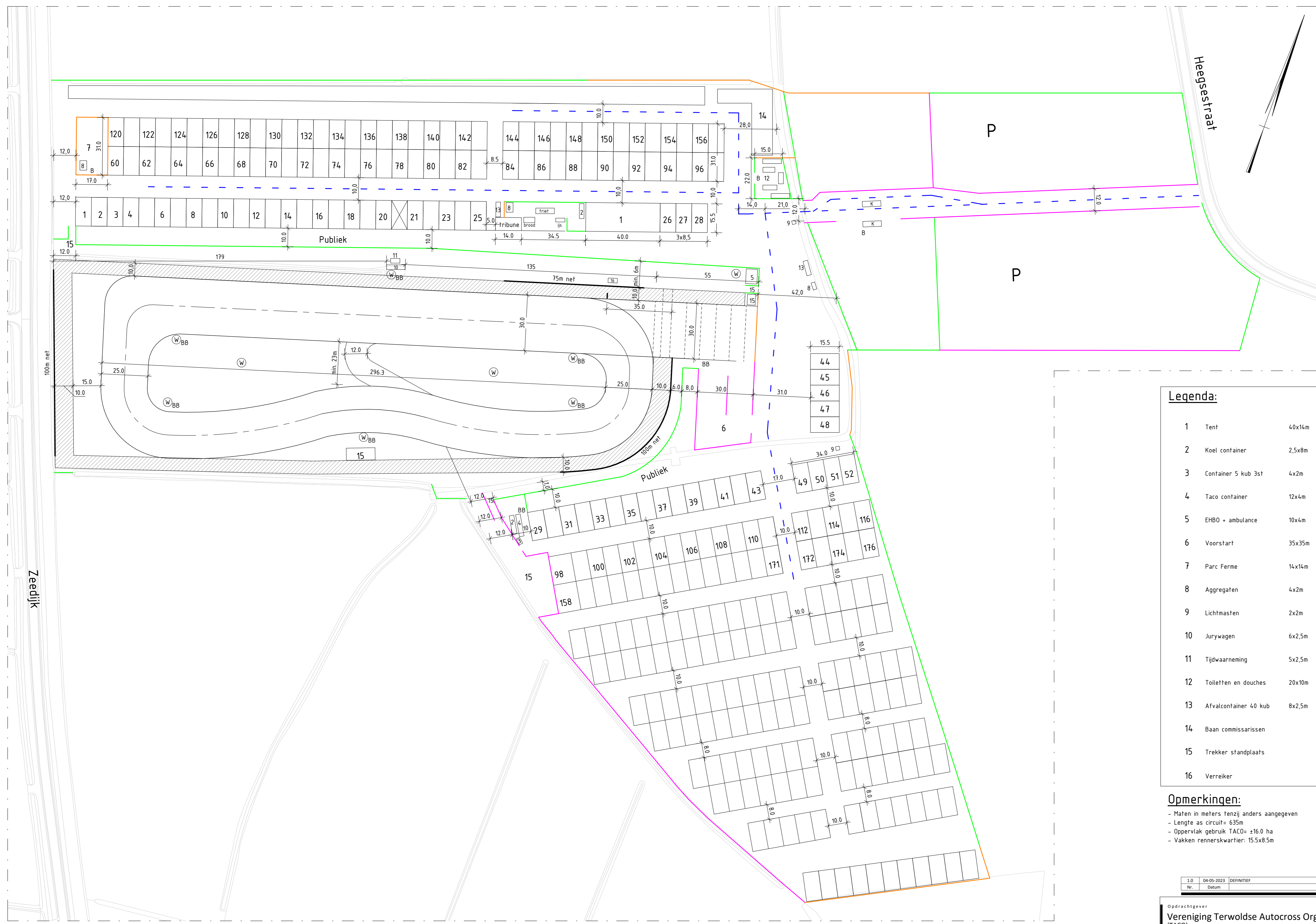
Bovenaanzicht Schaal: 1 : 1000
